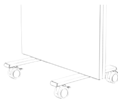
verrijdbare voet lengte: 50cm breedte: 6cm hoogte: 11cm
